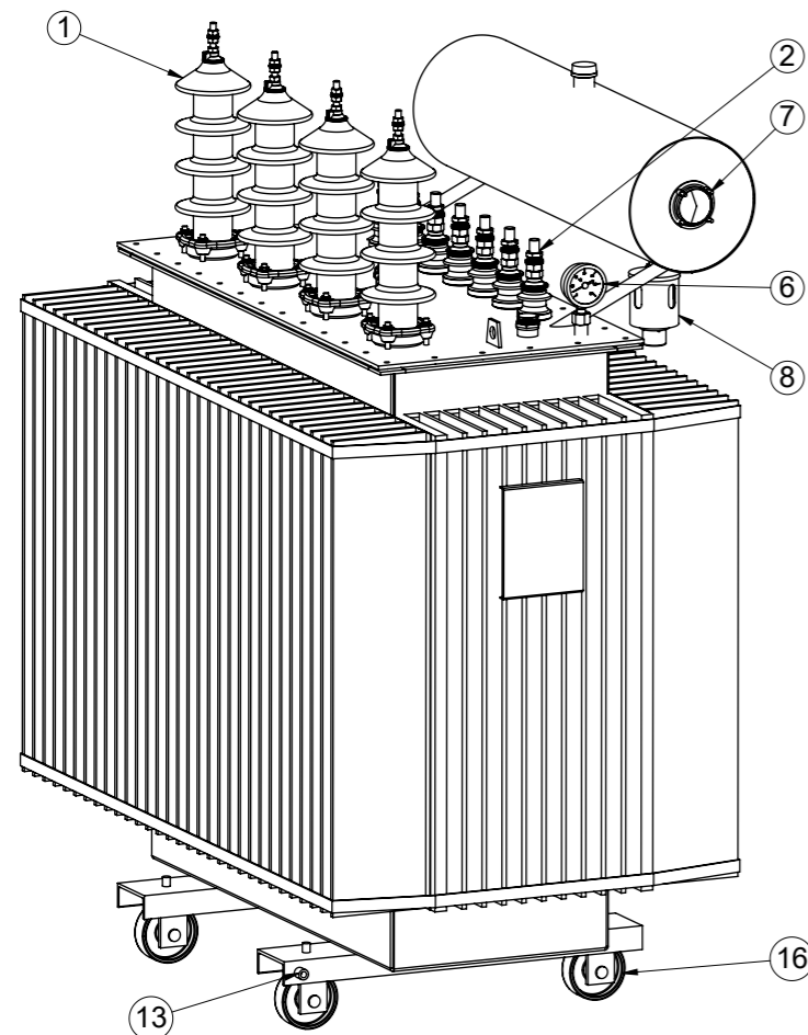
PERSPETIVA ISOMETRICA
